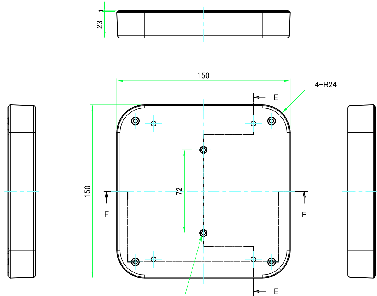
2-M4用インサートナット(ポールマウント WPMB-M4-2取付用) 2-M4 Insert nut for Pole mounting bracket (WPMB-M4-2)
